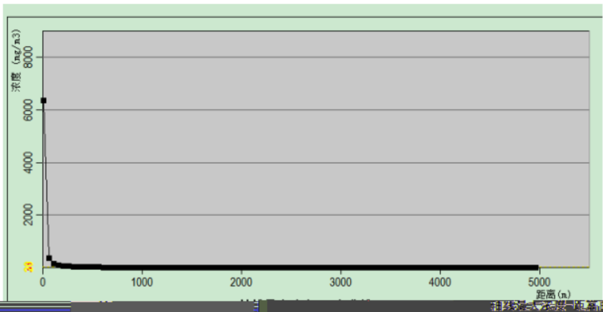
图3.4-1 最不利气象条件下氰化氢浓度距离变化曲线图
